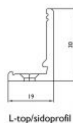
L-top/sidoprofil
