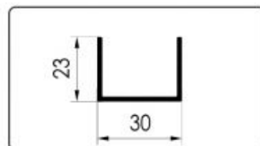
Anslagsprofil R304
