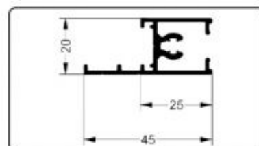
Fasglasprofil R109
