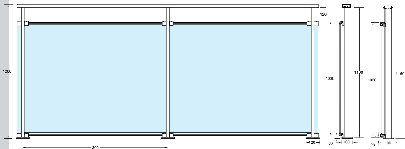
ELXIS TYP-A/B TOPPMONTERAD
