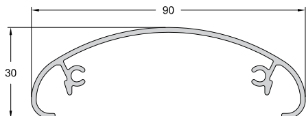
Täcklock för handledare 90x30
