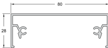
Lock för handledare 80x28
