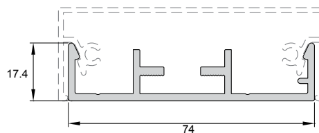
Underdel för handledare (744221/222)
