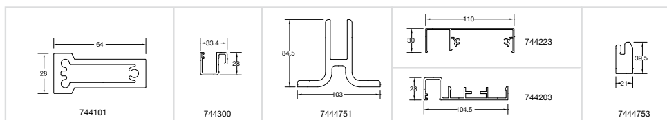
ELXIS SIDOMONTERING
